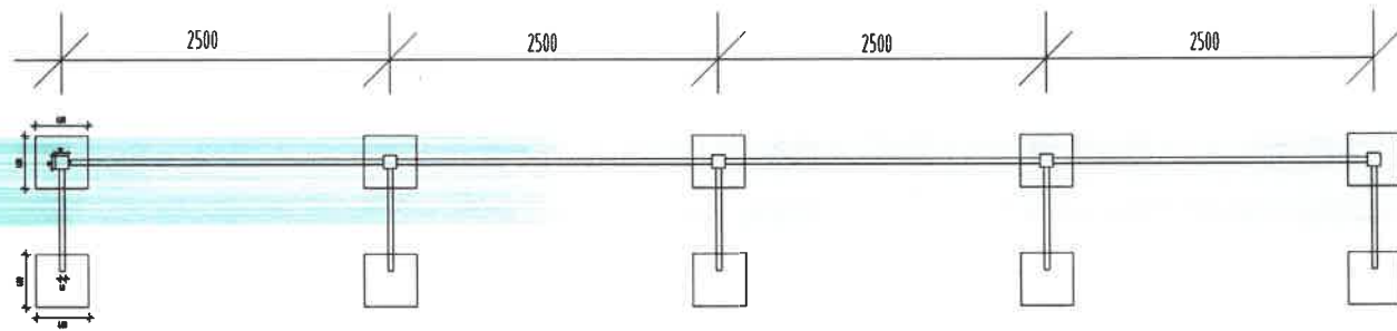
280 运输道路彩钢瓦护栏平面图
