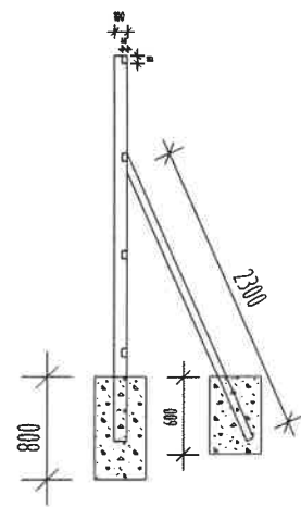
280 运输道路彩钢瓦护栏剖面图
