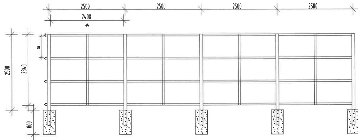
280 运输道路彩钢瓦护栏立面图
